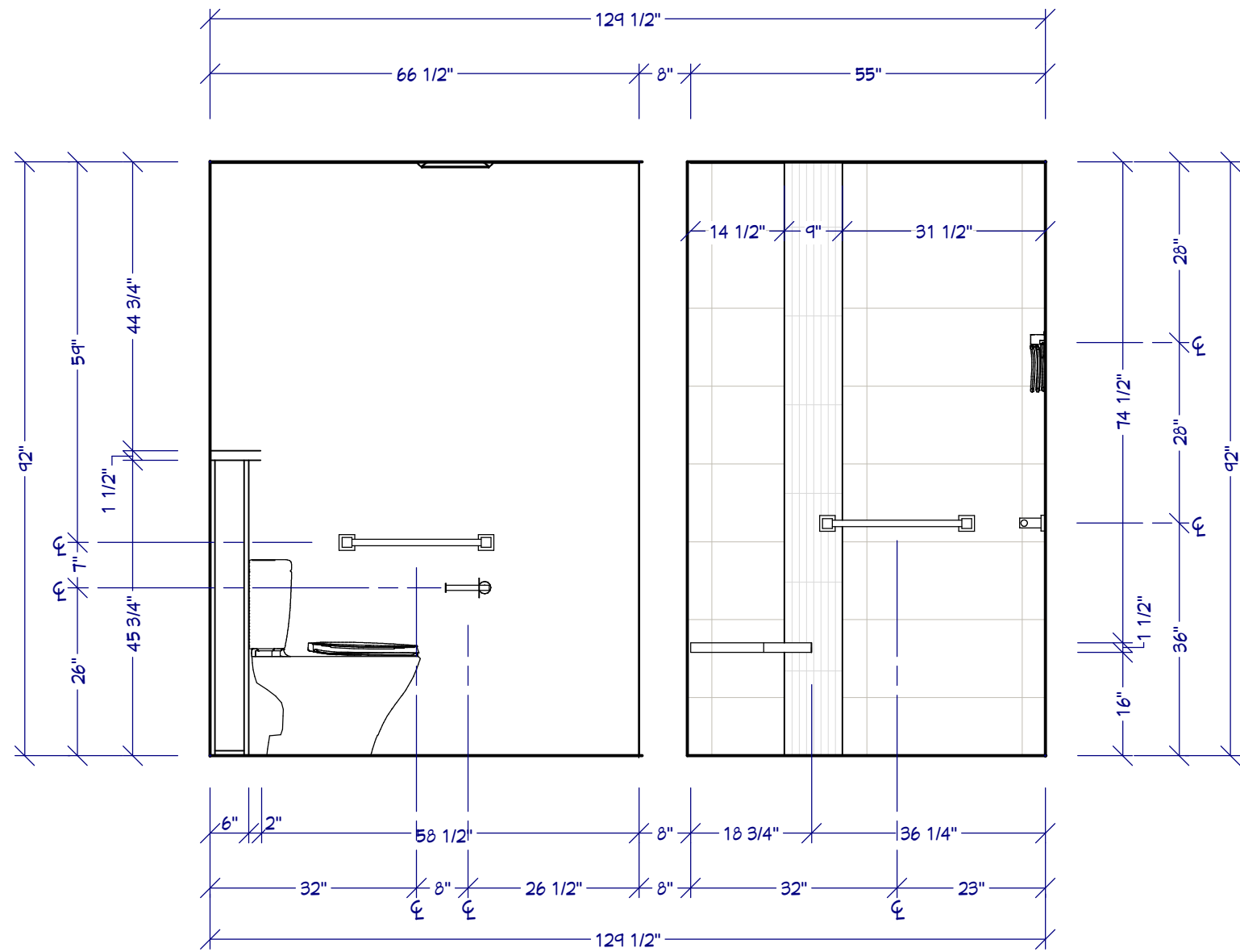
E ELEVATION E 1/2" = 1'
